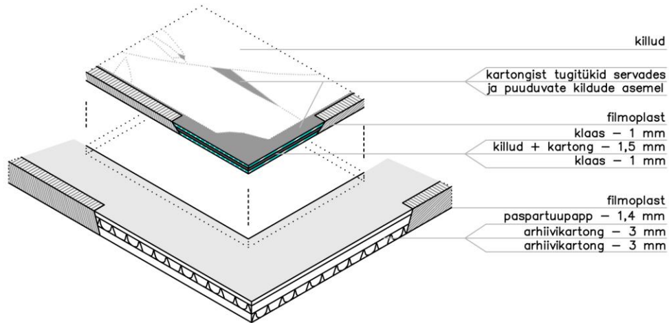
45. Läbilõige klaasfotode kildude jaoks kujundatud übristest koos kihtide paksustega (mm).
